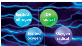
Elektróny sa zrážajú a zlučujú s dusíkom a kyslíkom vo vzduchu, čím vytvárajú 4 druhy nových zlúčenín.
