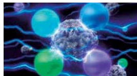
Tieto zlúčeniny majú vysokú oxidačnú schopnosť.
